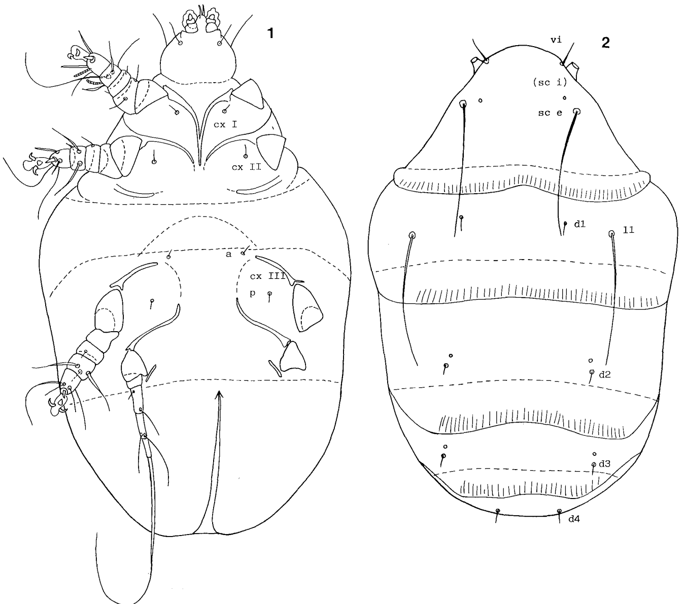
Figs. 1-2. Chrysolobobia elytrospherae n. sp. Femelle en vue ventrale (1) et dorsale (2).
