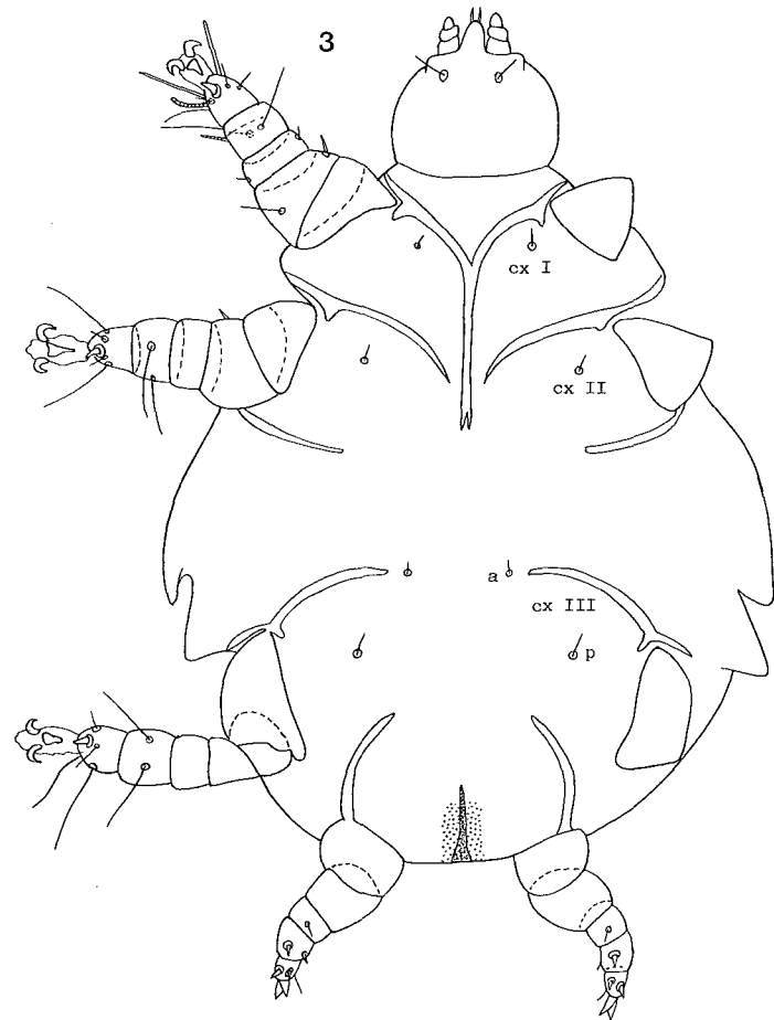
Fig. 3. Chrysomelobia elytrosphaerae n. sp. Male en vue ventrale.
