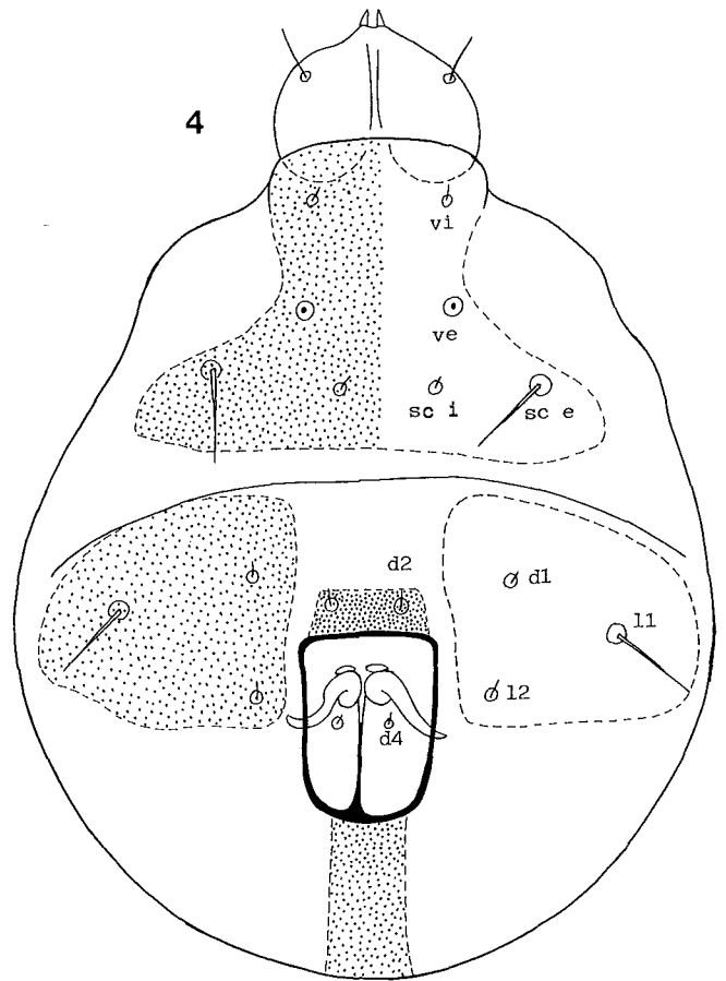
Fig. 4. Chrysomelobia elytrosphaerae n. sp. Male en vue dorsale.
