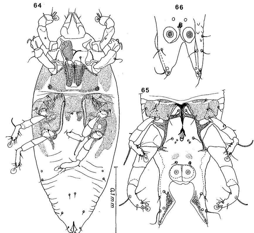
Fig. 64-66. — Oryzomysia longilobata FAIN. Allotype femelle (fig. 64) et holotype mâle (fig. 65 : hysterosoma) en vue ventrale. Oryzomysia peruviana boliviana ssp. n. Extrémité postérieure de l'holotype mâle en vue ventrale (fig. 66).
