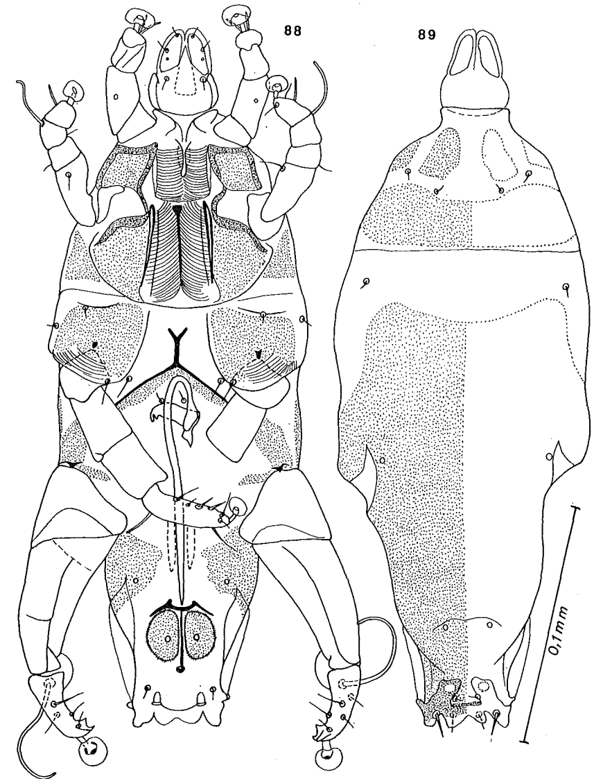
Fig. 88-89. — Prodidelphoecius euphallus FAIN. Holotype mâle en vue ventrale (fig. 88) et dorsale (fig. 89).
