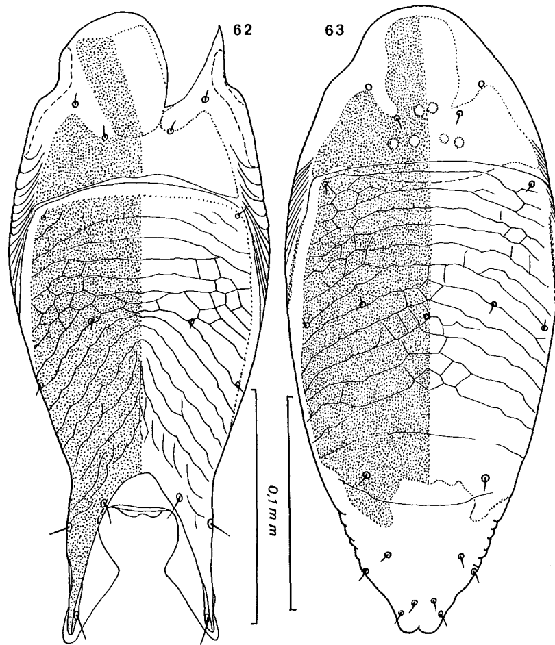
Fig. 62-63. — Oryzomysia longilobata FAIN. Holotype mâle (fig. 62) et allotype femelle (fig. 63) en vue dorsale.
