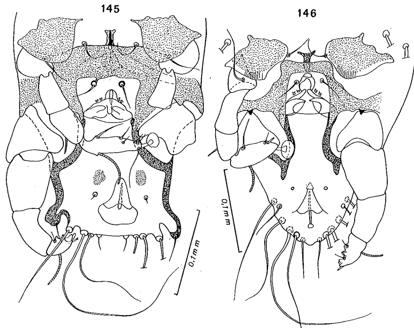
Fig. 145-146. — Listrocarpus surinamensis FAIN. Allotype mâle en vue ventrale (fig. 145 : hysterosoma). Listrocarpus cebi FAIN. Allotype mâle en vue ventrale (fig. 146 : hysterosoma).
