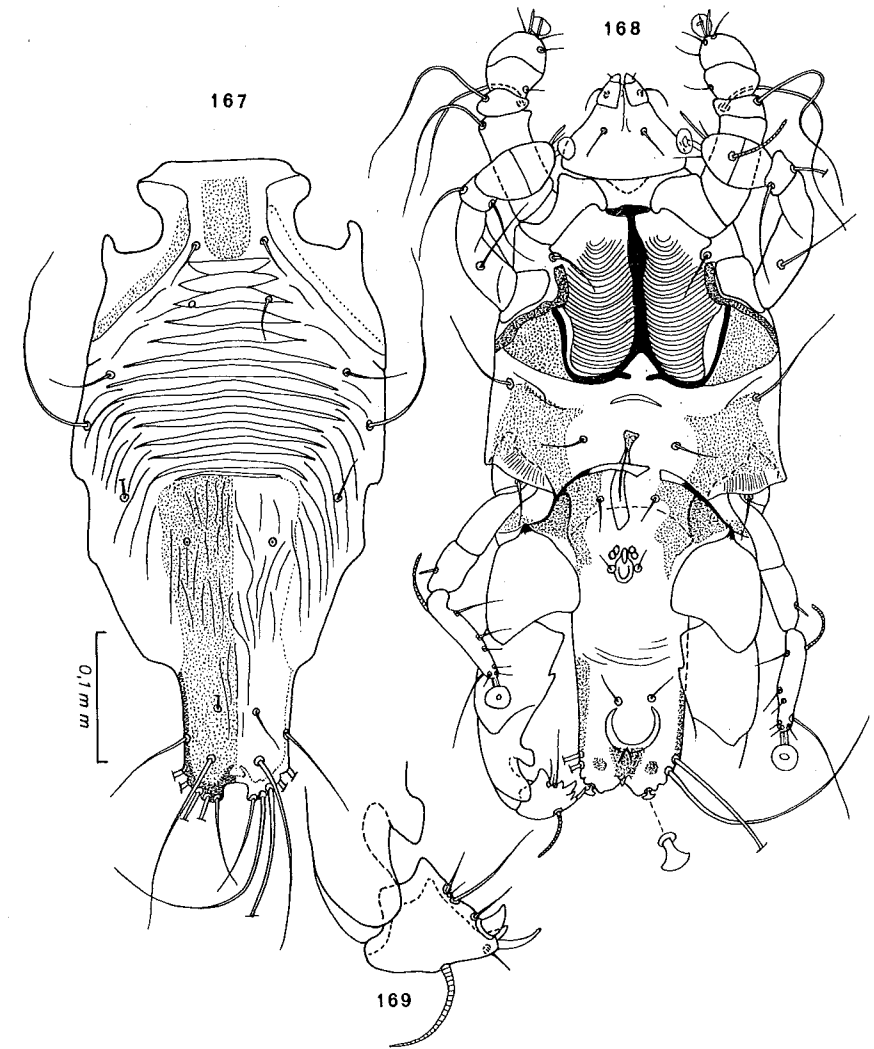
Fig. 167-169. — Capromysia elongata (FAIN). Holotype mâle en vue dorsale (fig. 167) et ventrale (fig. 168); tibiotarse IV (fig. 169).
