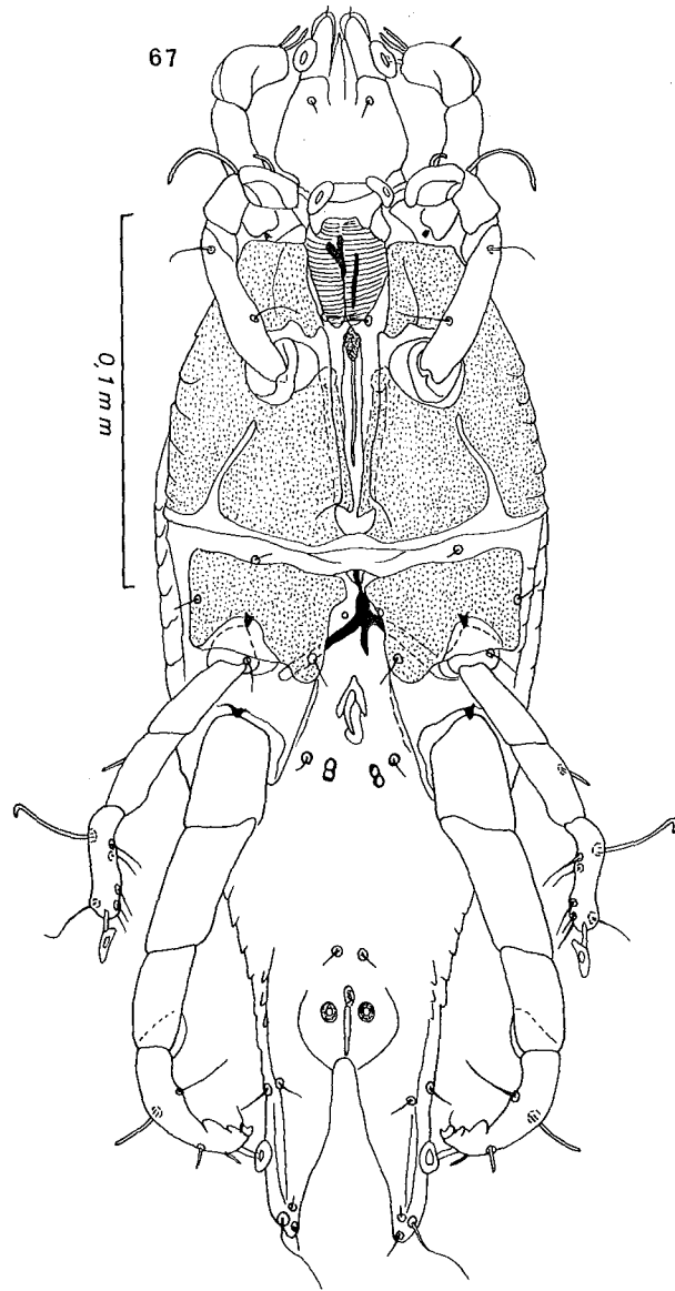
Fig. 67. — Oryzomyia peruviana FAIN. Holotype mâle en vue ventrale.
