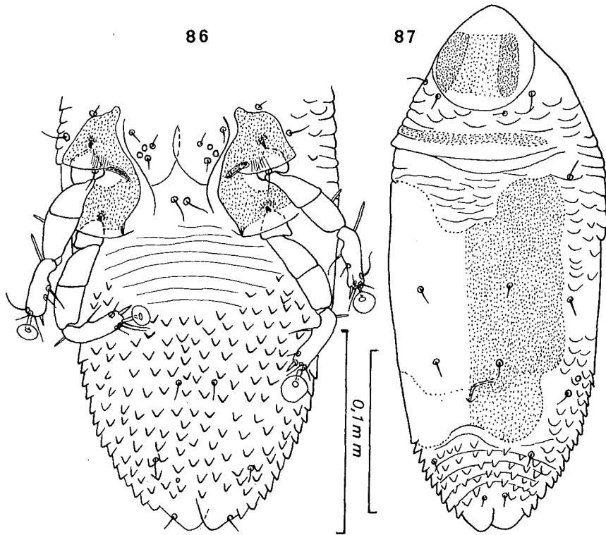
Fig. 86-87. — Dromichiolichus chiliensis FAIN. Allotype femelle en vue ventrale (fig. 86 : hysterosoma) et dorsale (fig. 87).
