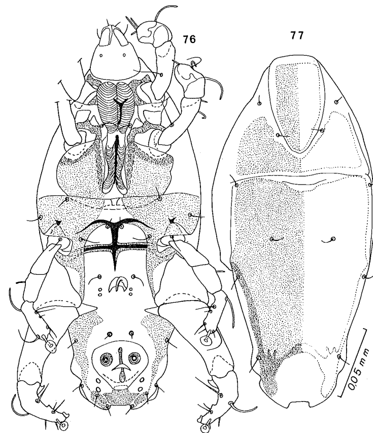
Fig. 76-77. — Oryzomyia oxymycterus FAIN. Allotype mâle en vue ventrale (fig. 76) et dorsale (fig. 77).
