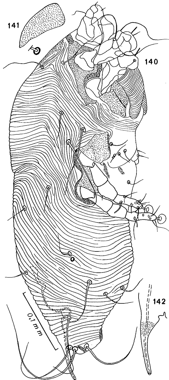
Fig. 140-142. — Listrocarpus hapalei FAIN. Holotype femelle vu latéralement (fig. 130); écusson postscapulaire chez un paratype (fig. 141); tube copulateur (fig. 142).
