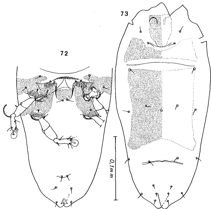
Fig. 72-73. — Oryzomysia oryzomys (RADFORD). Paralectotype femelle en vue ventrale (fig. 72) et dorsale (fig. 73).
