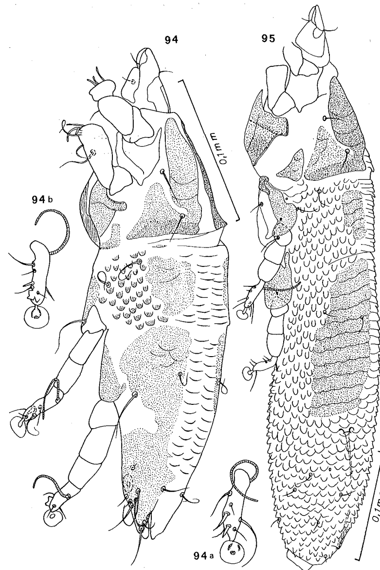
Fig. 94-95. — Didelphoecius philander FAIN. Holotype mâle en vue latérale (fig. 94); tarse III (fig. 94a) et IV (fig. 94b) chez un paratype.
