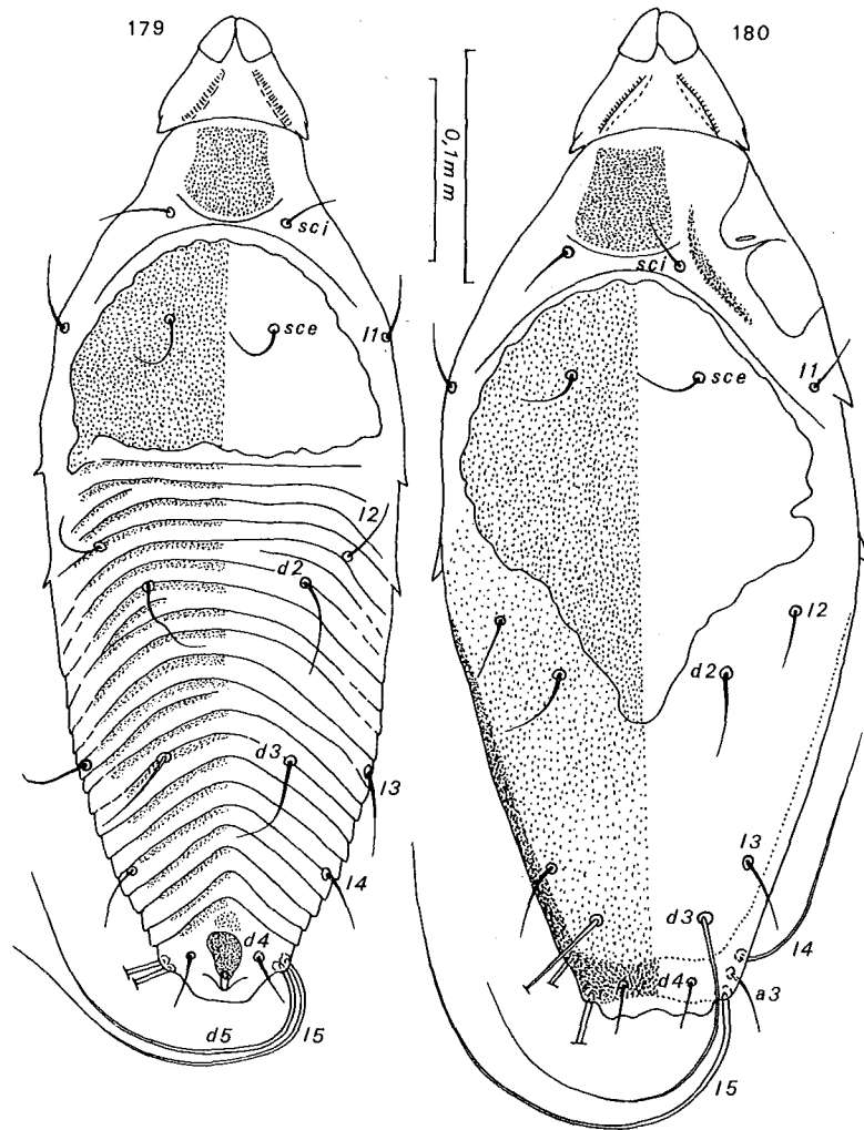
Fig. 179-180. — Domingoecius cruzi FAIN et LUKOSCHUS, sp. n. Face dorsale de l'holotype femelle (fig. 179) et de l'allotype mâle (fig. 180).
