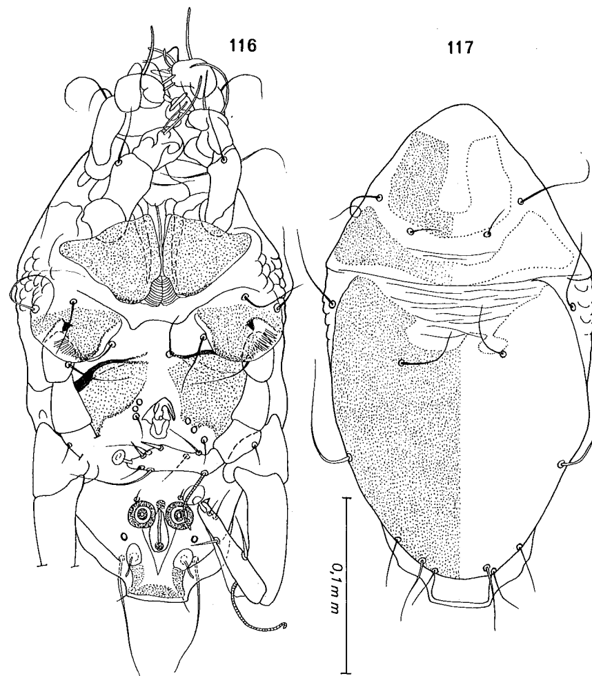
Fig. 116-117. — Didelphoecius scutatus FAIN. Mâle en vue ventrale (fig. 116) et dorsale (fig. 117) (dessins d'après l'holotype et un paratype).
