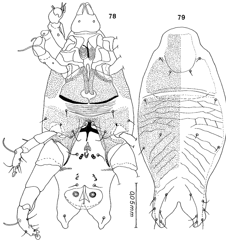
Fig. 78-79. — Oryzomyia lukoschusi FAIN. Holotype mâle en vue ventrale (fig. 78) et dorsale (fig. 79).
