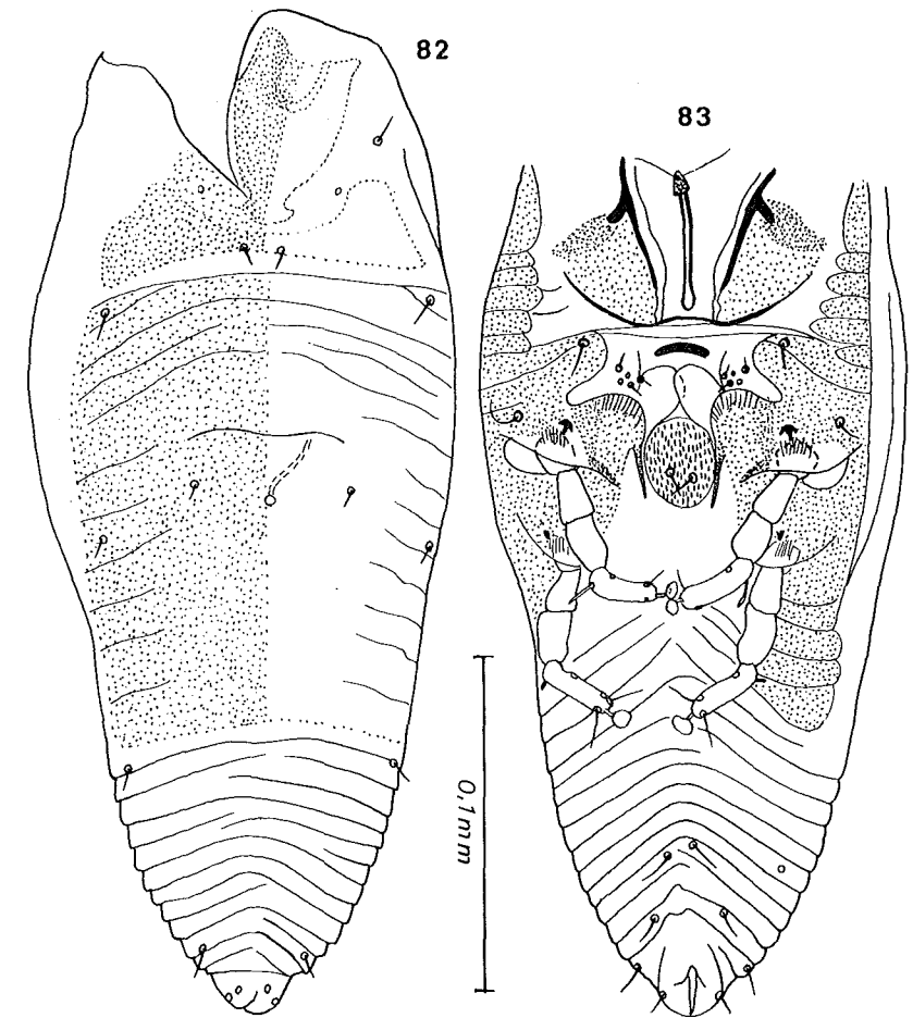
Fig. 82-83. — Oryzomyia striata sp. n. Holotype femelle en vue dorsale (fig. 82) et ventrale (fig. 83).
