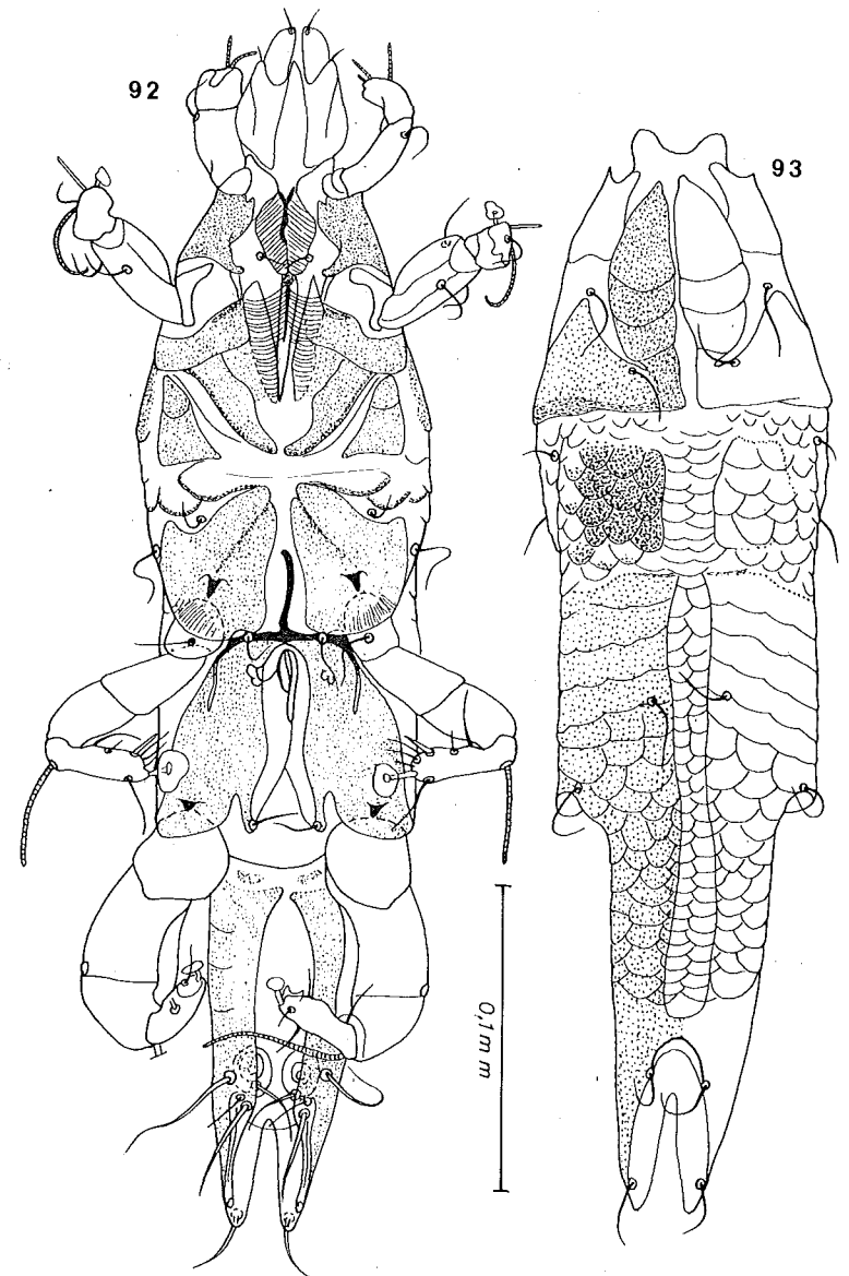
Fig. 92-93. — Didelphoecius colombianus manaoensis ssp. n. Holotype mâle en vue ventrale (fig. 92) et dorsale (fig. 93).
