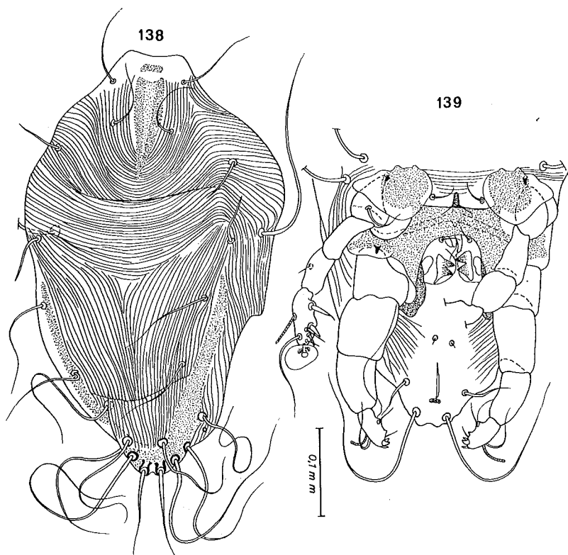
Fig. 138-139. — Listrocarpus lagothrix FAIN. Allotype mâle en vue dorsale (fig. 138) et ventrale (fig. 139 : hysterosoma).
