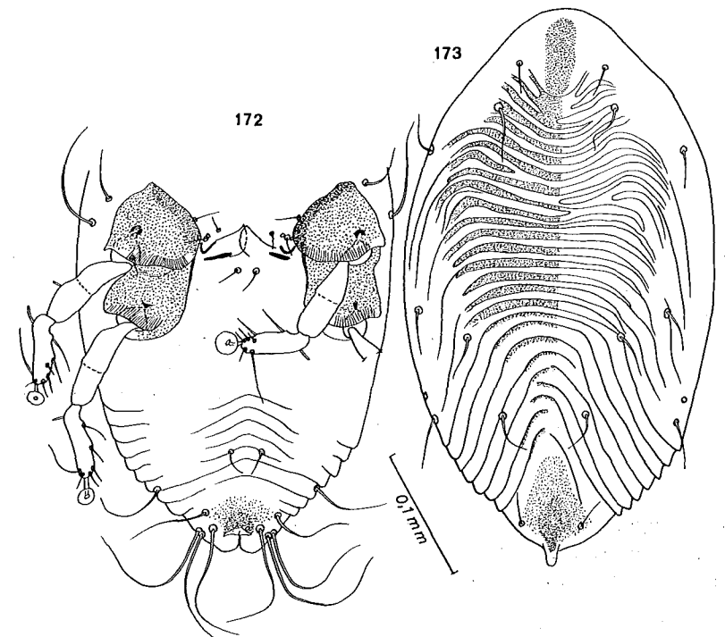
Fig. 172-173. — Capromylichus cubanus FAIN. Allotype femelle en vue ventrale (fig. 172 : hysterosoma) et dorsale (fig. 173).
