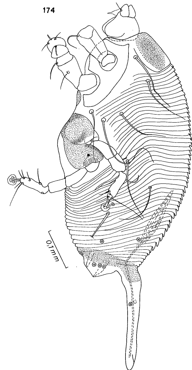
Fig. 174. — Plagiodontochirus nudus FAIN. Femelle en vue latérale (dessin d'après l'holotype et les paratypes).
