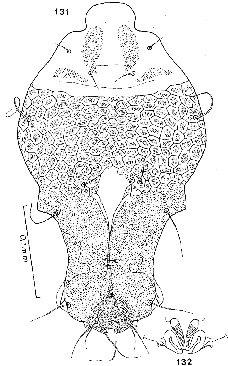
Fig. 131-132. — Didelphilichus serrifer FAIN. Holotype mâle vu dorsalement (fig. 131); détail des organes postaux (fig. 132).
