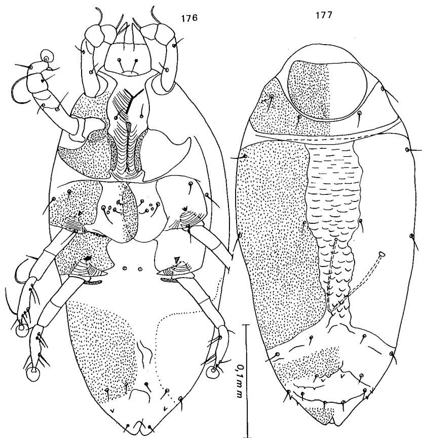
Fig. 176-177. — Euryzygomysia catharinae sp. n. Femelle holotype, en vue ventrale (fig. 176) et dorsale (fig. 177).
