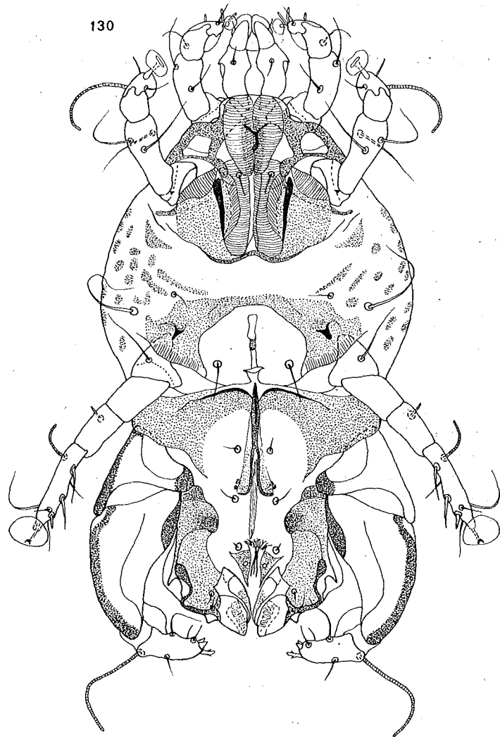
Fig. 130. — Didelphilichus serrifer FAIN. Holotype mâle vu ventralement.
