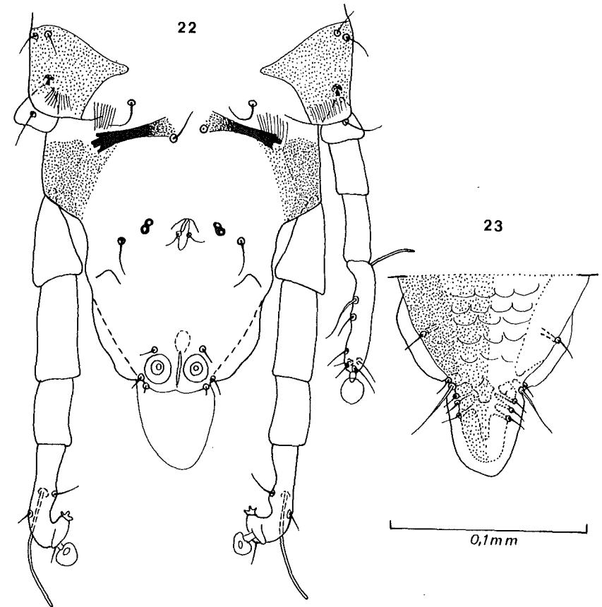
Fig. 22-23. — Chirodiscoides interruptus FAIN. Holotype mâle. Hysterosoma en vue ventrale (fig. 22) et extrémité postérieure du corps en vue dorsale (fig. 23).
