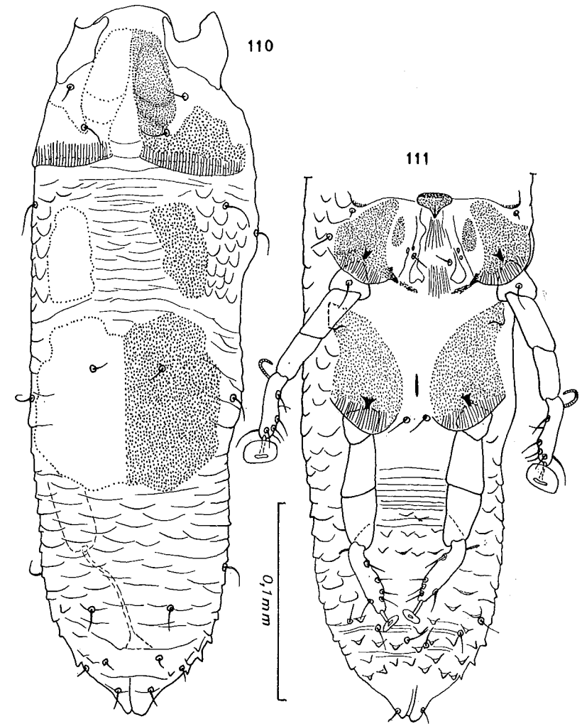
Fig. 110-111. — Didelphoecius callipygus FAIN. Allotype femelle en vue dorsale (fig. 110) et ventrale (fig. 111 : hysterosoma).
