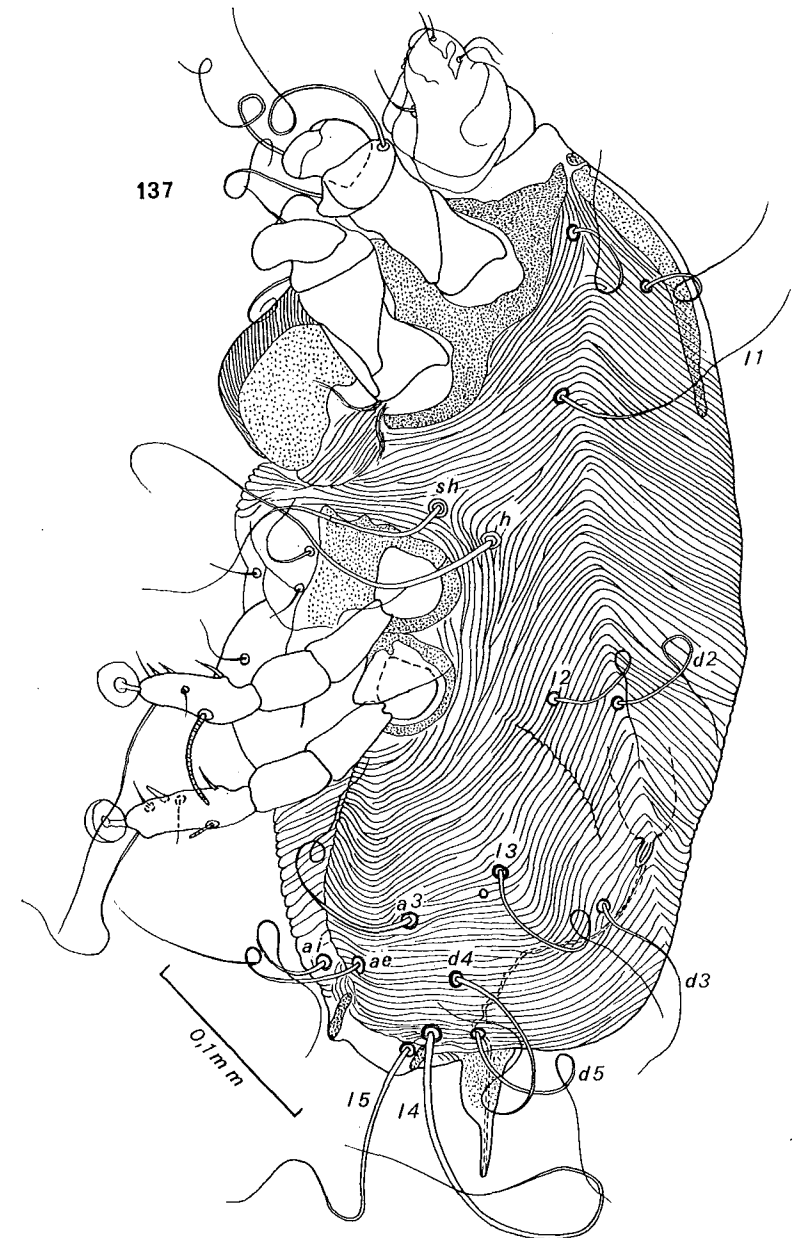
Fig. 137. — Listrocarpus lagothrix FAIN. Holotype femelle vu latéralement.
