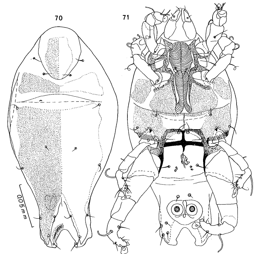
Fig. 70-71. — Oryzomysia oryzomys (RADFORD). Lectotype mâle en vue ventrale (fig. 70) et dorsale (fig. 71).
