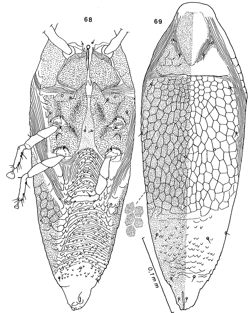
Fig. 68-69. — Oryzomyia peruviana FAIN. Allotype femelle en vue ventrale (fig. 68) et dorsale (fig. 69).
