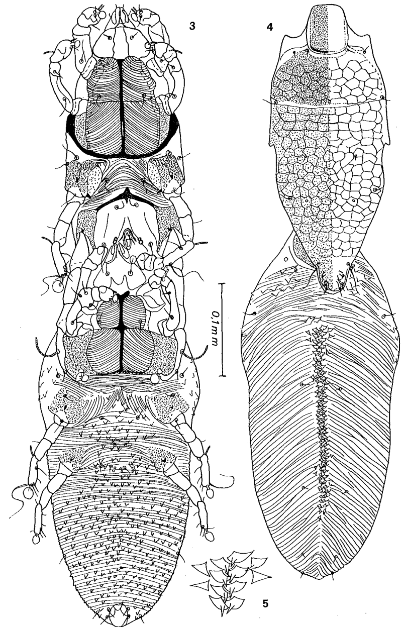
Fig. 3-5. — Chirodiscoides caviae HIRST. Mâle accouplé avec une tritonymphe femelle en vue ventrale (fig. 3) et dorsale (fig. 4). Détail des écailles médiadorsales de la tritonymphe femelle (fig. 5).
