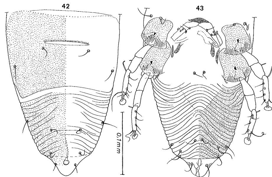
Fig. 42-43. — Isothricola appendiculatus FAIN. Allotype femelle : hysterosoma en vue dorsale (fig. 42) et ventrale (fig. 43).
