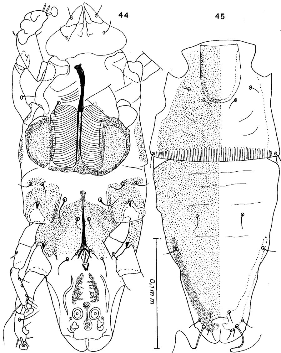
Fig. 44-45. — Isothricola amazonicus FAIN. Holotype mâle en vue ventrale (fig. 44) et dorsale (fig. 45).
