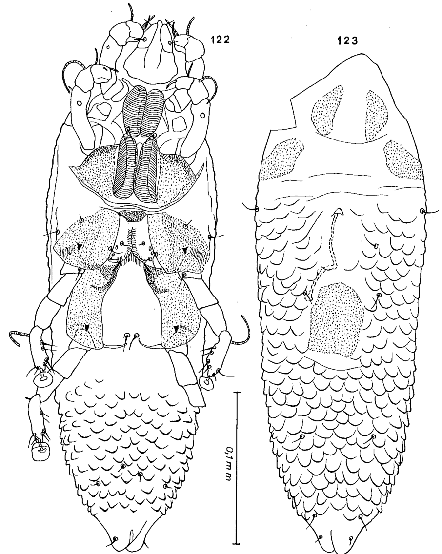
Fig. 122-123. — Didelphoecius paranensis FAIN. Allotype femelle en vue ventrale (fig. 122) et dorsale (fig. 123).
