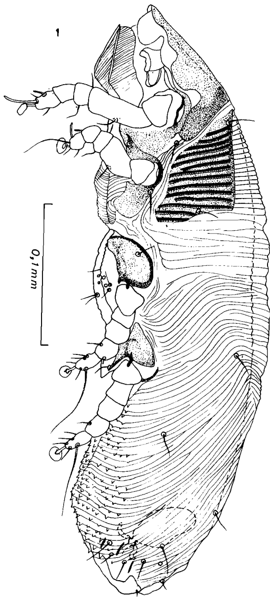
FIG. 1. — Listrophorus occitanus n.sp. Holotype femelle
