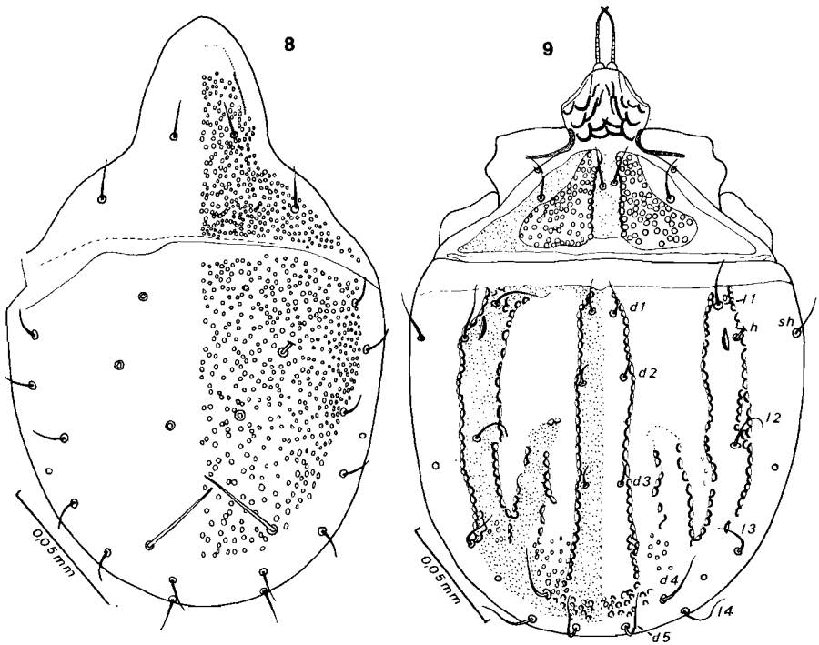
FIG. 8-9 : Face dorsale des hypopes de Chiloanoetus mayumbensis sp.n. (fig. 8) et de Curculanoetus rhynchophorus sp.n. (fig. 9).
