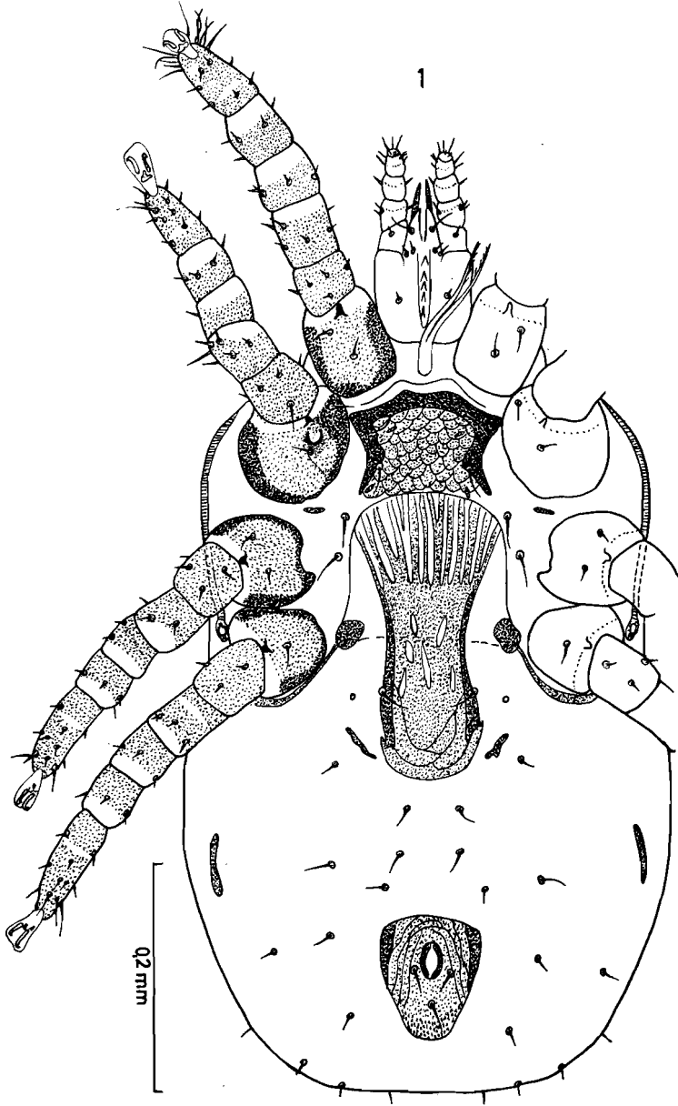
FIG. 1. — Hemilaelaps liobeterodon sp.n. Femelle en vue ventrale
