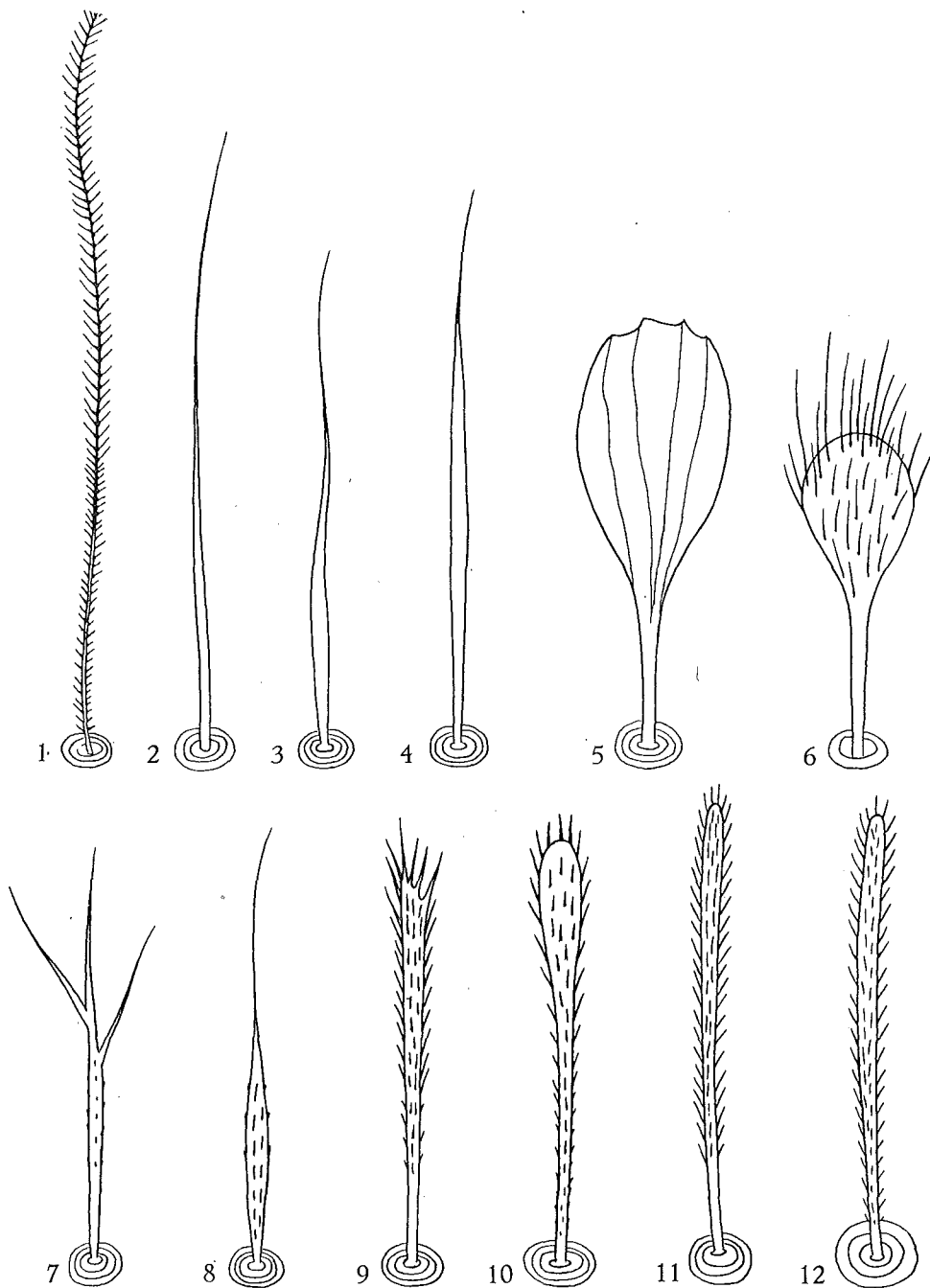
Fig. 1-12. — Sensillae chez Ereynetoides watsoni (1); Lawrencarus eweri (2); Speleognathus bovis (holotype ♀) (3); Neospeleognathopsis chiropteri (holotype ♀) (4); N. bastini (paratype ♀) (5); N. duboisi (holotype ♀) (6); Paraspeleognathopsis bakeri (holotype ♀) (7); P. galagoensis (holotype ♀) (8); P. strandtmanni (allotype ♀) (9); P. galliardi (holotype ♀) (10); P. derricki (♀) (11); P. ruandae (holotype ♀) (12).
