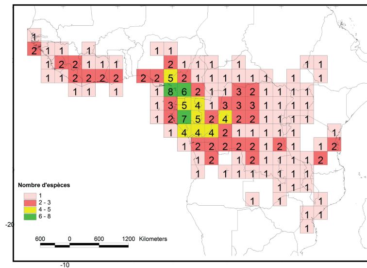
Fig. 73. Richesse spécifique générale du genre Craterispermum (les chiffres indiquent le nombre total d'espèces présentes dans chaque maille de 2,5° × 2,5°).
