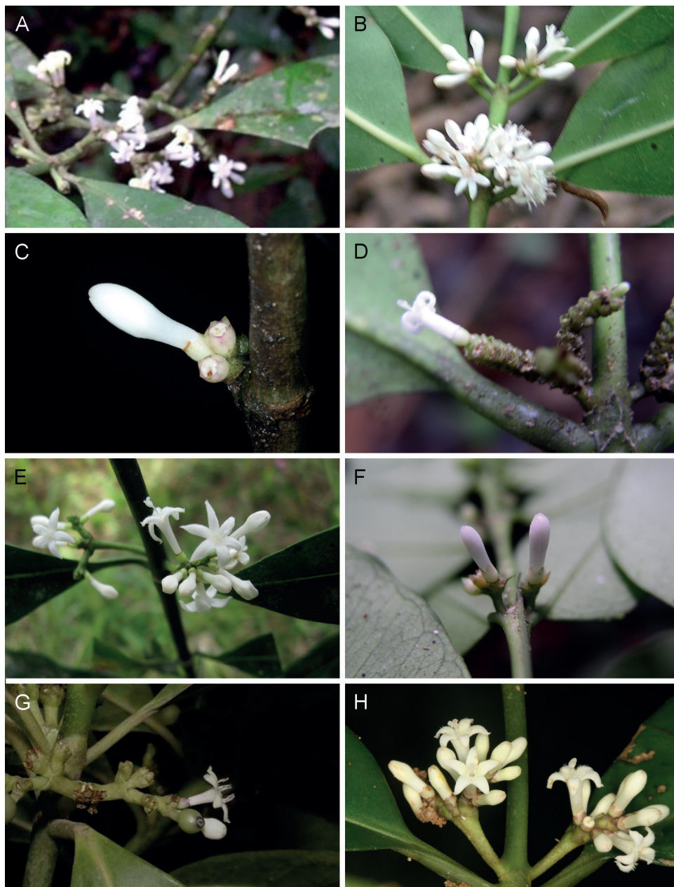
Fig. 12. Quelques inflorescences observées dans le genre Craterispermum . A. C. ledermannii . B. C. schweinfurthii . C. C. rumpianum . D. C. robbrechtianum . E. C. cerinanthum . F. C. parvifolium . G. C. laurinum . H. C. ledermannii var. modestum . (Crédits photographiques : A = Droissart, V. ; B, E = Taedoumg, H. ; C = Dessein, S. ; D, F = Simo, M. ; G = Birnbaum, P. ; H = Stévert, T.)
